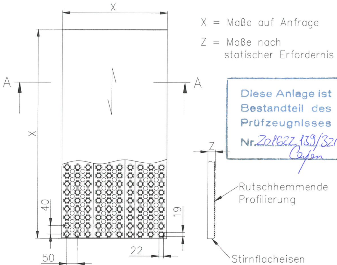
Schnitt A-A
