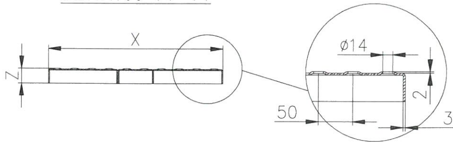
Schnitt A-A
